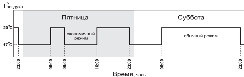
Рис.7 График температуры воздуха в помещении для Режима 3.
