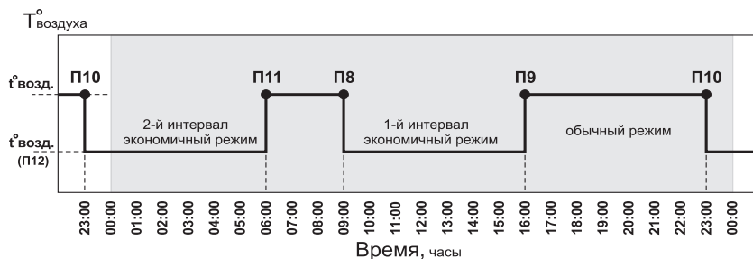
Рис.5 График температуры воздуха в помещении для Режимы 1.
