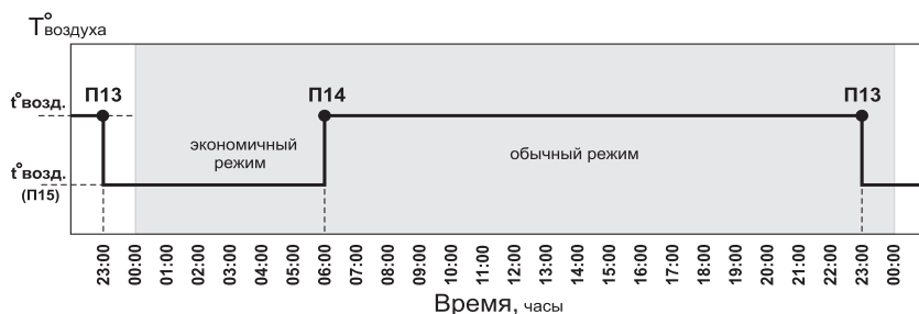
Рис.6 График температуры воздуха в помещении для Режимы 2.
